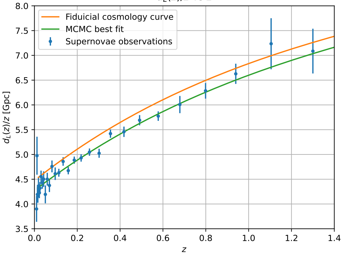
d_L(z)/z vs z
